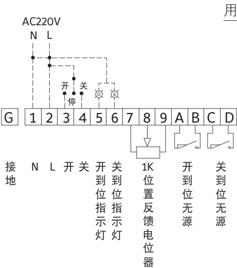
图4：开关型执行器(型号带BDC)接线图
