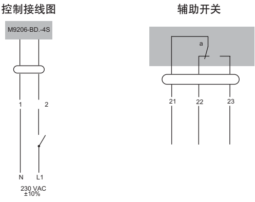
M9206-BDx-4S接线图
