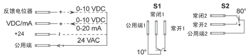
M9106-GGx-4接线图
