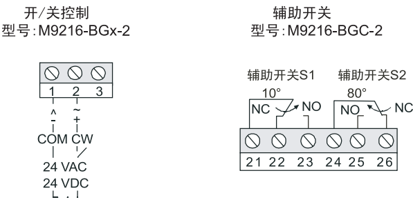
M9216-BGx-2接线图
