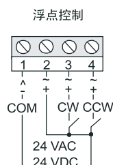
控制接线图 型号: M9216-AGx-2
