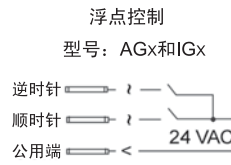
M9106-AGx-4接线图
