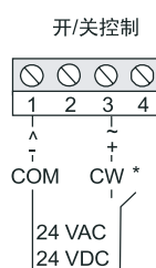
M9216-AGx-2接线图
