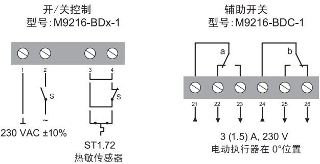
M9216-BDx-1接线图
