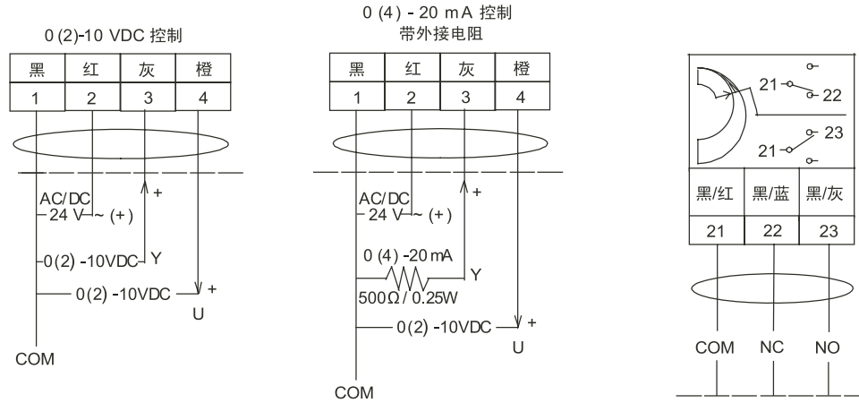
M9206-GGx-4S接线图
