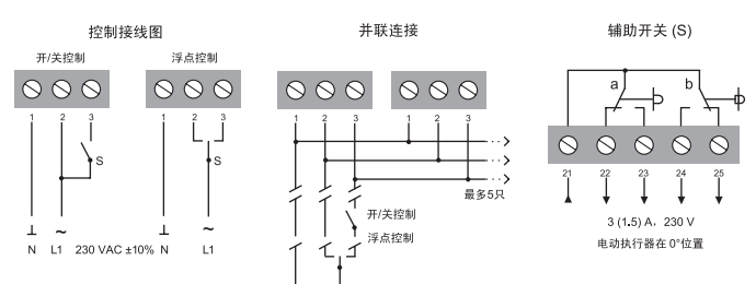
M9108 ADx 1接线图
