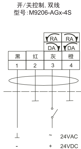
M9206-AGx-4S接线图
