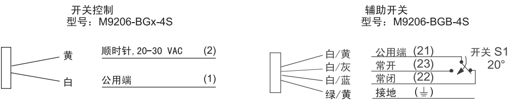
M9206-BGx-4S接线图
