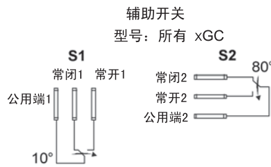
M9109 AGx 4接线图
